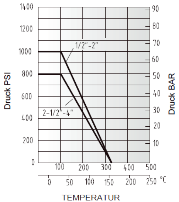
Drucktemperaturbewertung 1/2"~4"
